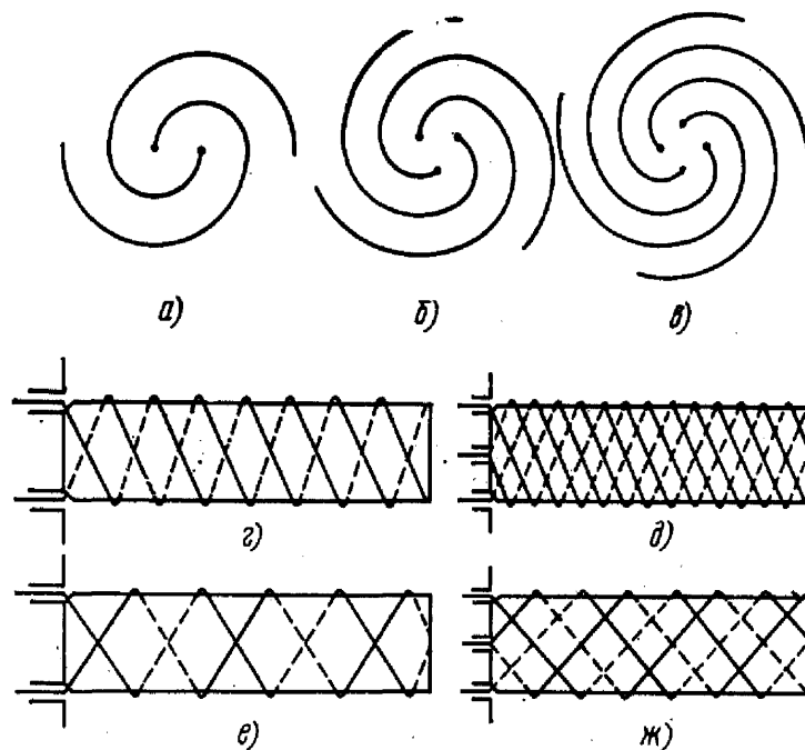
Рис. 3.3. Многозаходные спиральные антенны
