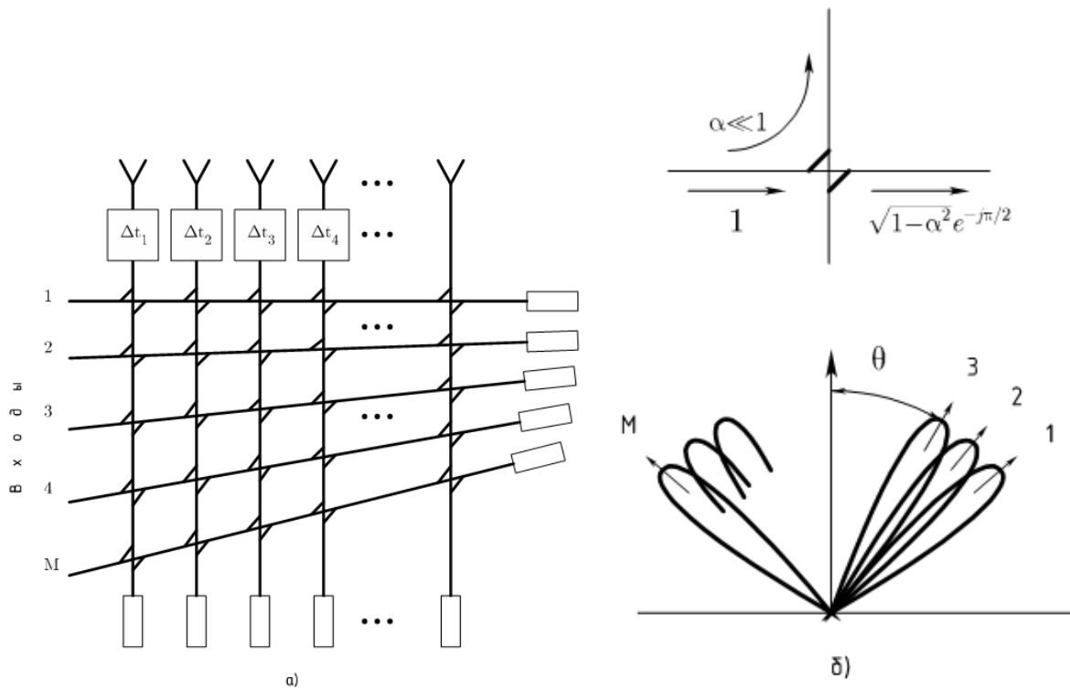
Рис. 10.7. Многолучевая антенная решетка с последовательным питанием
