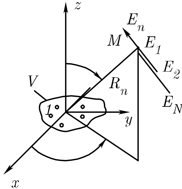
Рис. 9.1. Пространство излучателей
