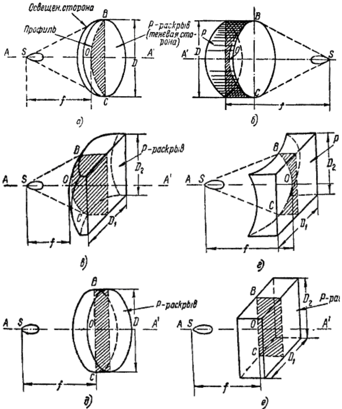
Рис. 5.2. Линзовые антенны:
