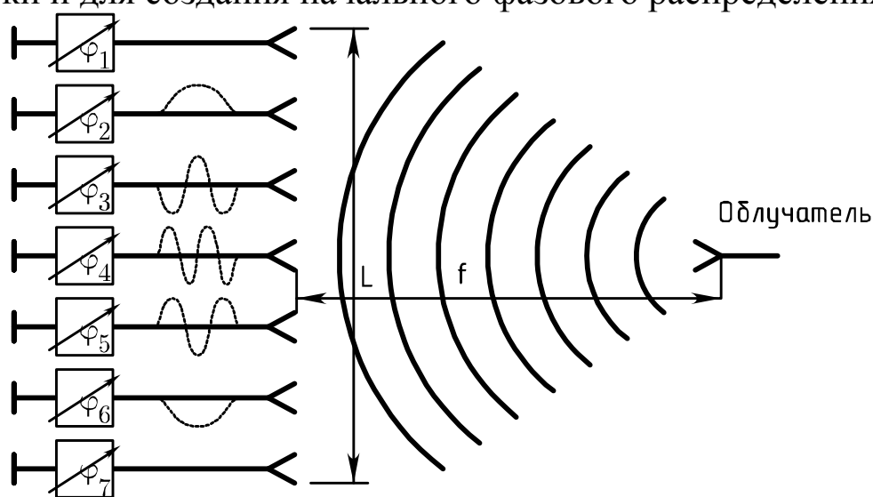
Рис. 10.5. Отражательная схема оптического питания излучателей
