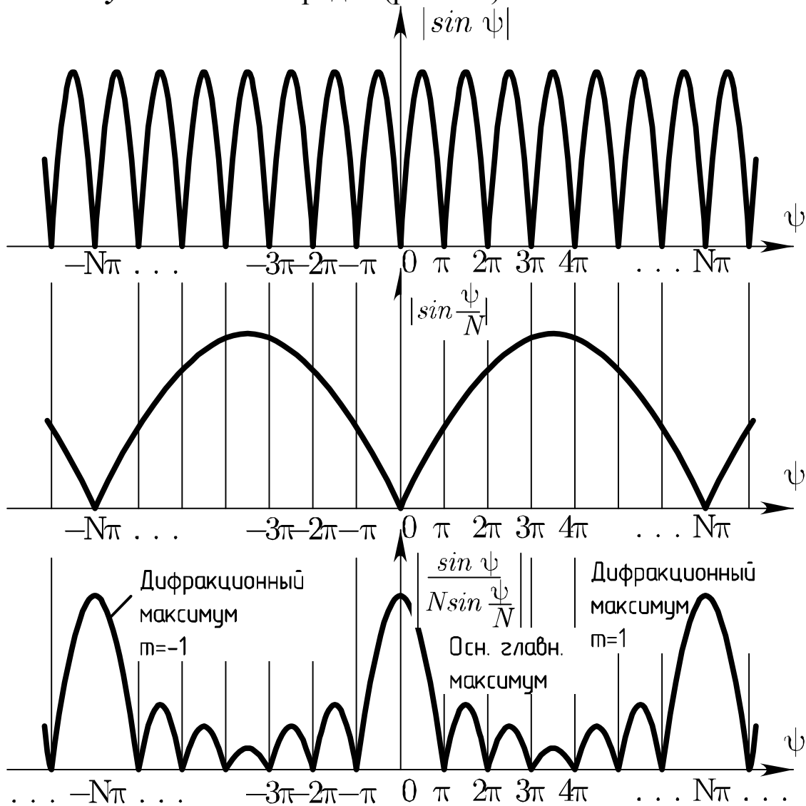
Рис. 9.3. Максимумы нормированной характеристики направленности решетки
