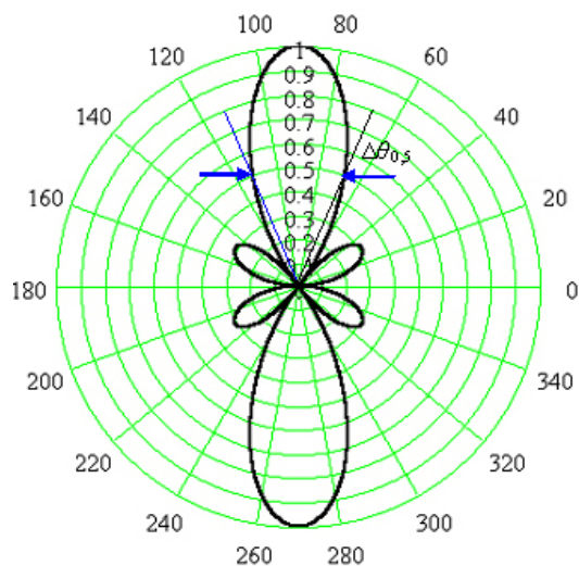
Рис. 1.2. ДН в полярных координатах
