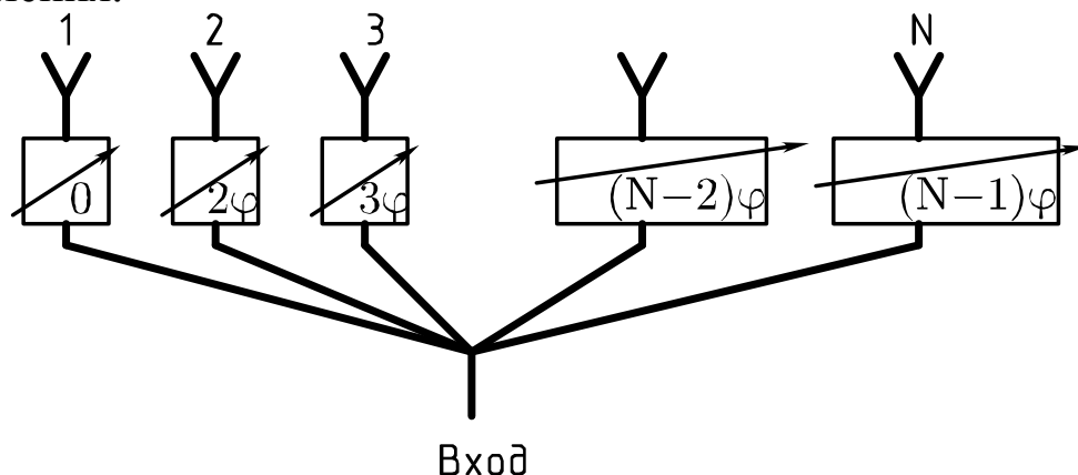
Рис. 10.2. Схема параллельного питания излучателей ФАР
