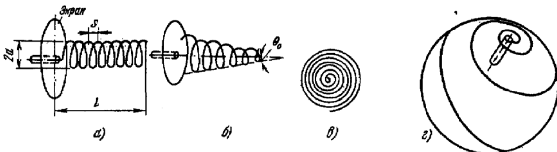
Рис. 3.1. Разновидности спиральных антенн
