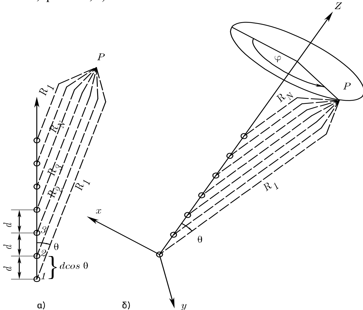
Рис. 9.2. Эквидистантная линейная решетка
