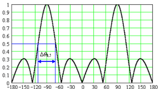
Рис. 1.3. ДН в декартовых координатах
