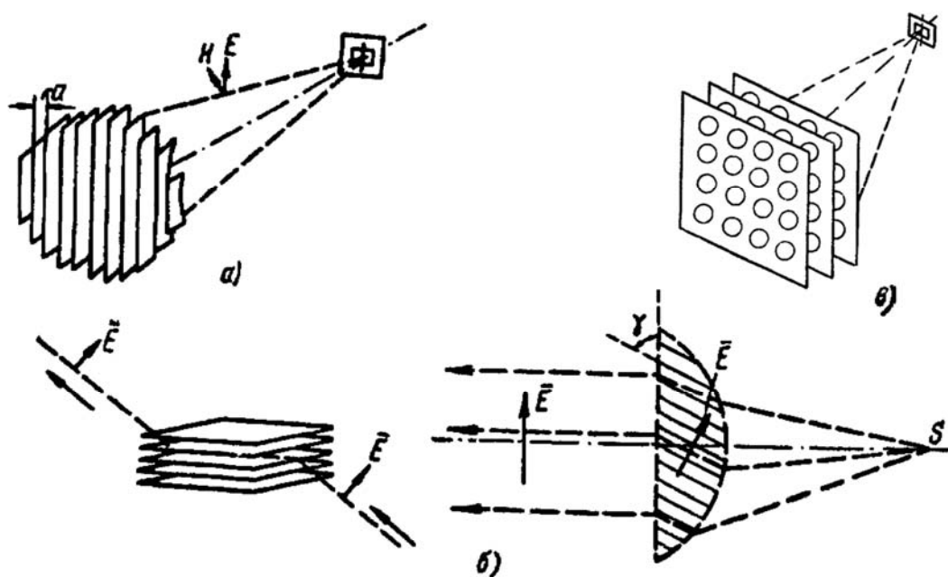
Рис. 5.3. Металлические линзы:
