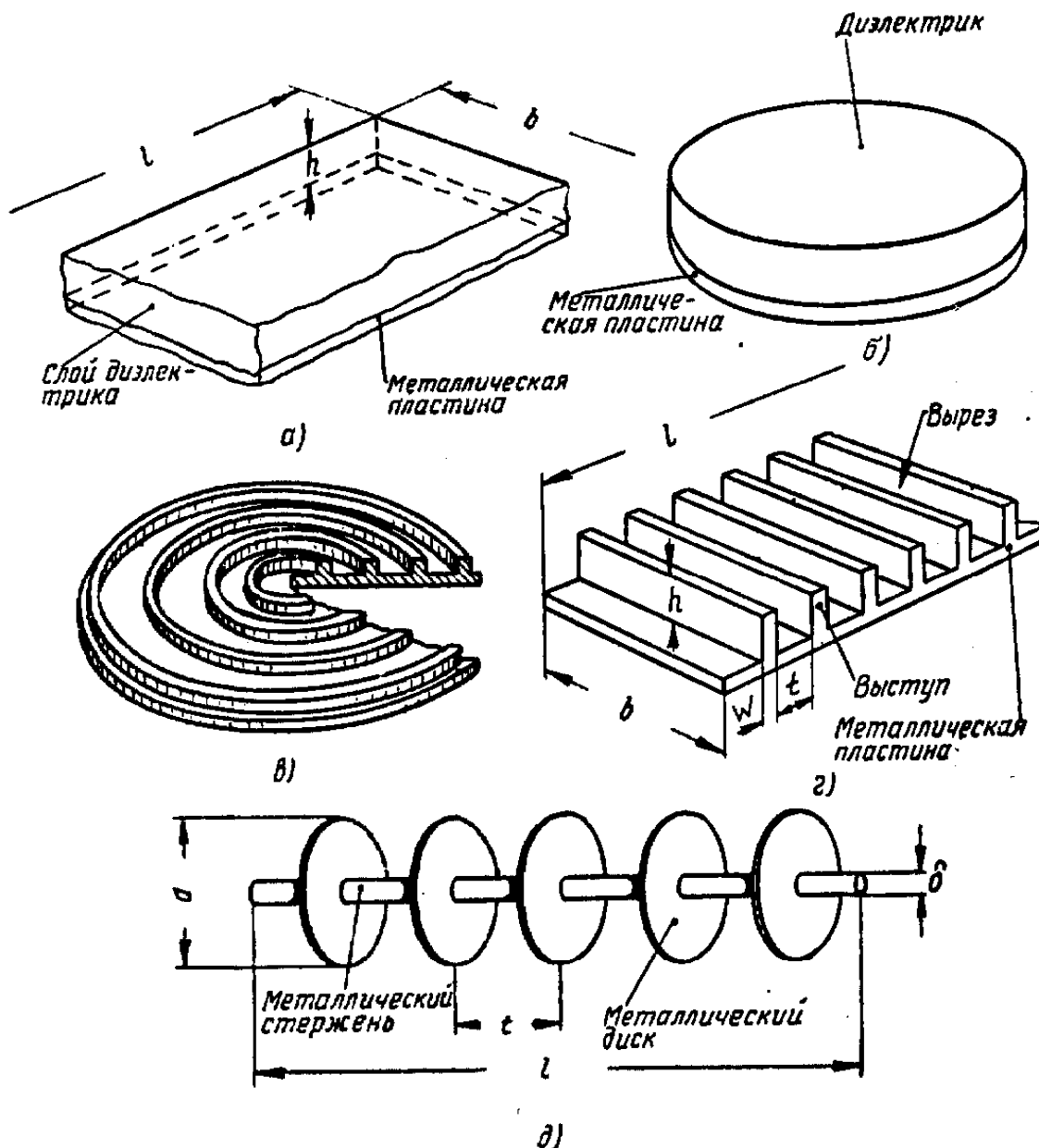
Рис. 7.1. Антенны поверхностных волн:
