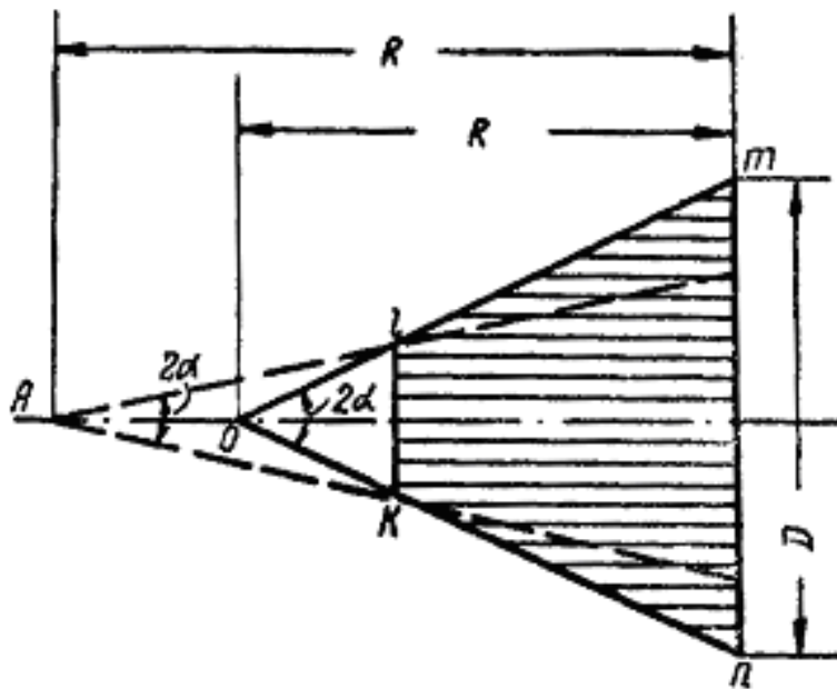
Рис. 4.2. Продольное сечение рупора
