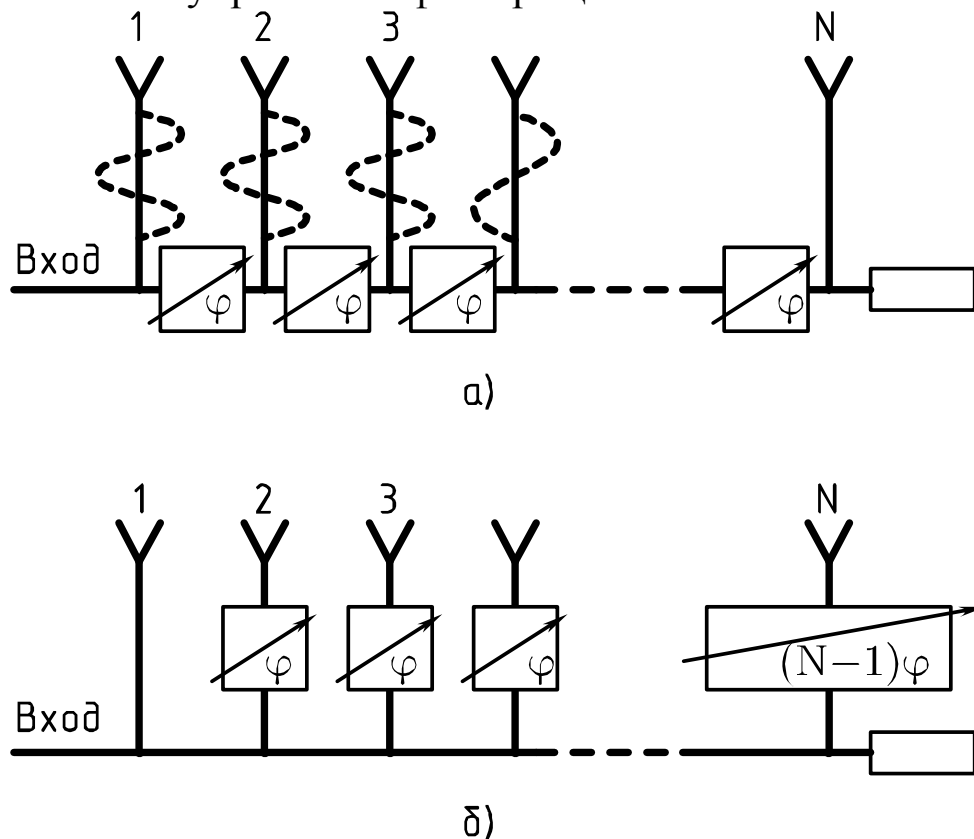
Рис. 10.1. Схема последовательного питания излучателей ФАР
