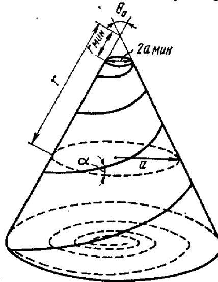
Рис. 3.2. Коническая спираль
