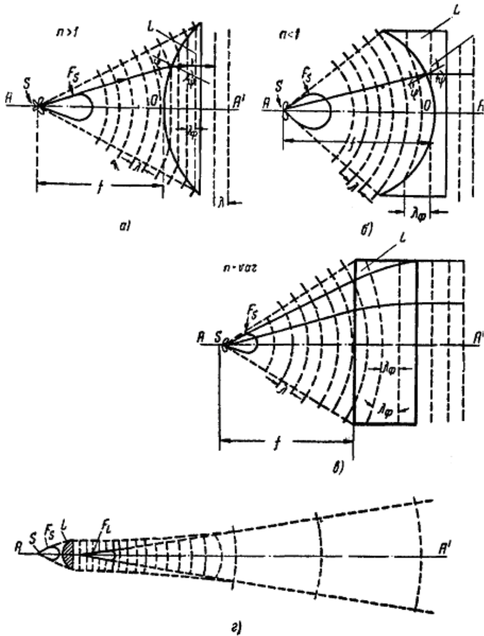
Рис. 5.1. Изменение формы волны линзовой антенной (в продольном сечении) при различных коэффициентах преломления n : а – при постоянном коэффициенте n > 1 (выпуклая, замедляющая линза); б – при постоянном коэффициенте n < 1 (вогнутая, ускоряющая линза); в – при переменном коэффициенте n (плоская линза); г – явление дифракции, вызывающее изменение формы волны на большом расстоянии от линзовой антенны
