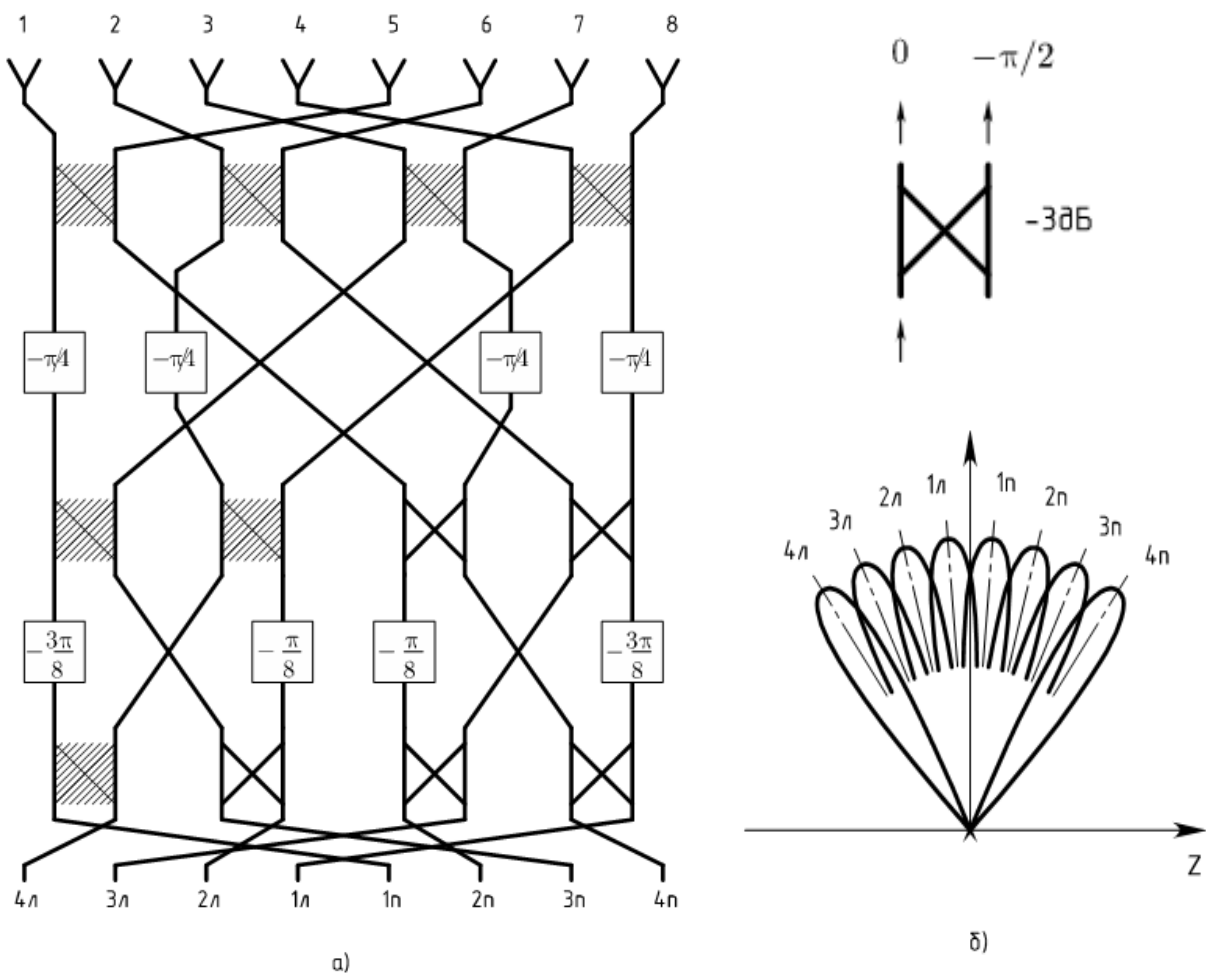
Рис. 10.8. Многолучевая антенная решетка с параллельным питанием
