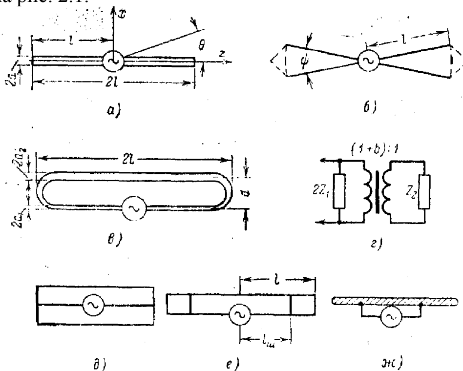
Рис. 2.1. Симметричные вибраторы:
