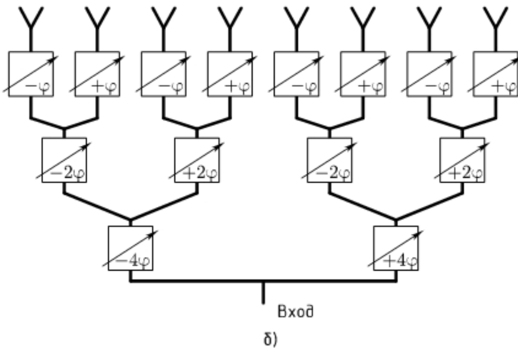
Рис. 10.3. Двоично-этажная схема питания излучателей ФАР
