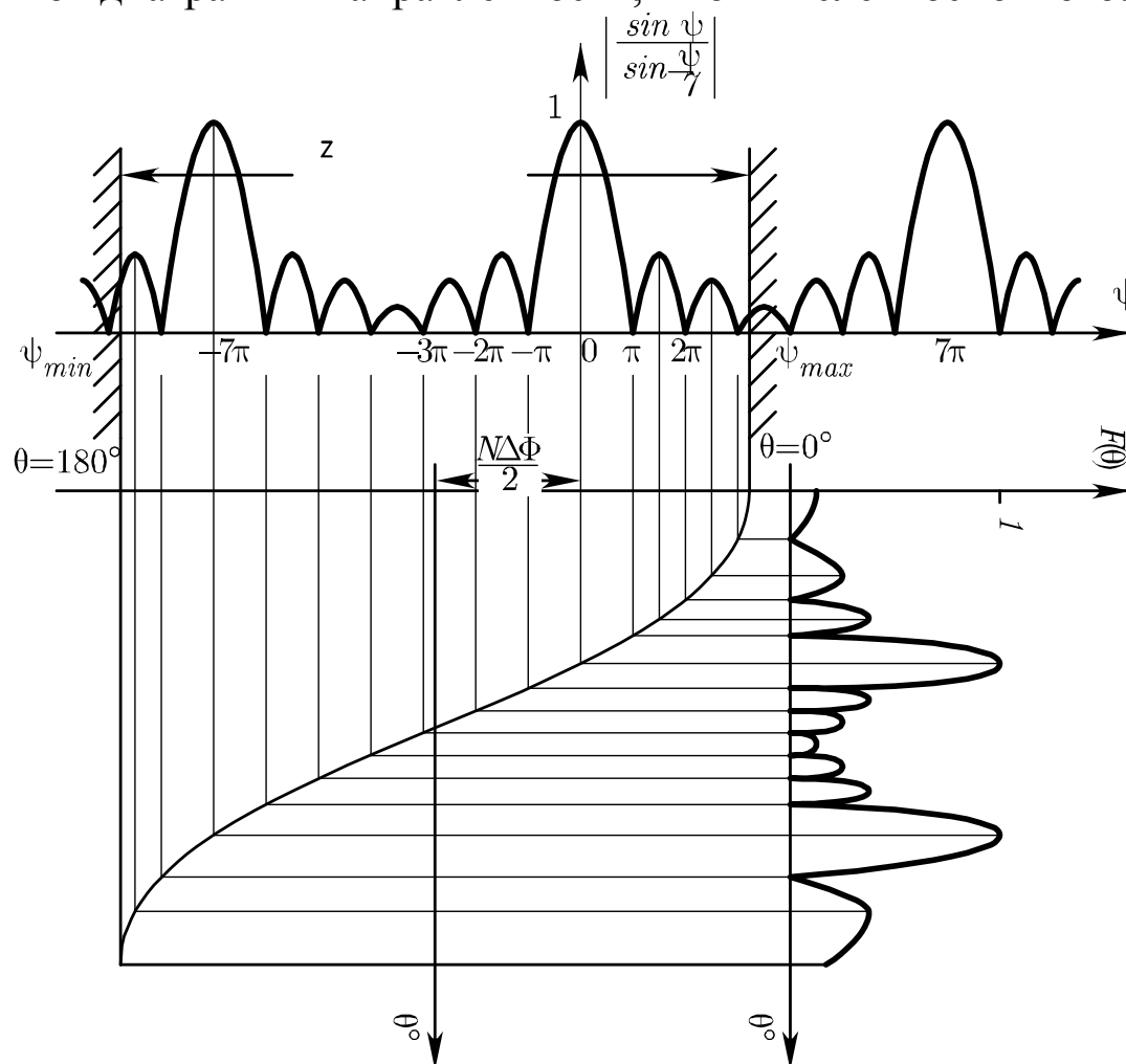
Рис. 9.4. К определению диаграммы направленности решетки
