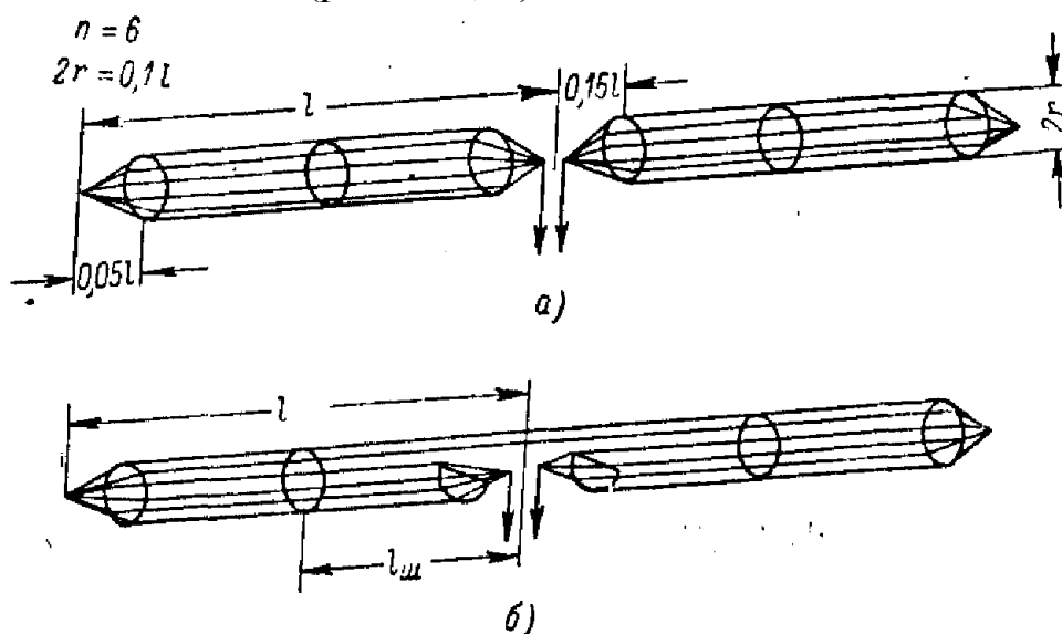
Рис. 2.2. Диполь Надененко:
