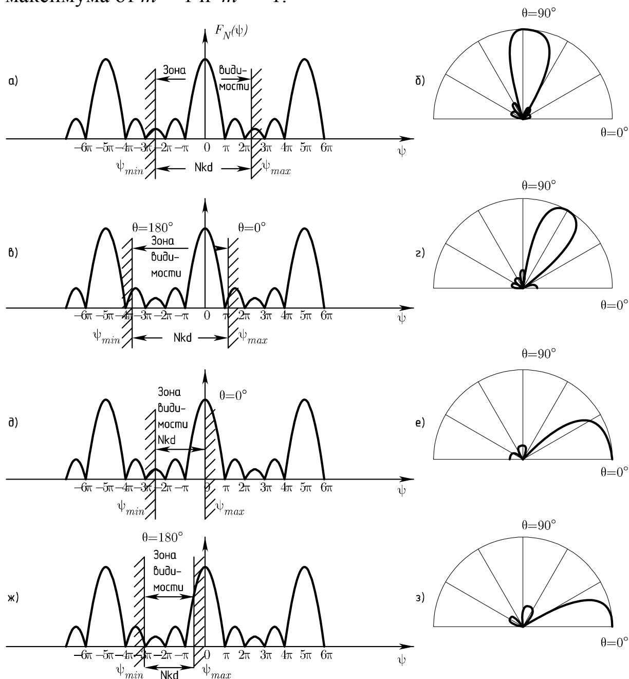
Рис. 9.6. Диаграмма направленности излучателя – щели при возбуждении ускоренной волной
