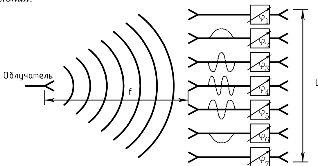
Рис. 10.4. Прходная схема оптического питания излучателей ФАР
