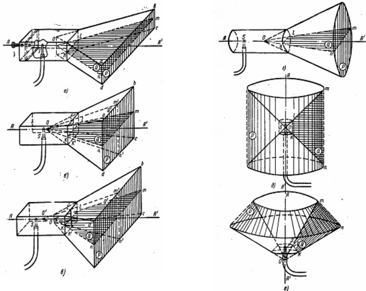
Рис. 4.1. Рупорные антенны:
