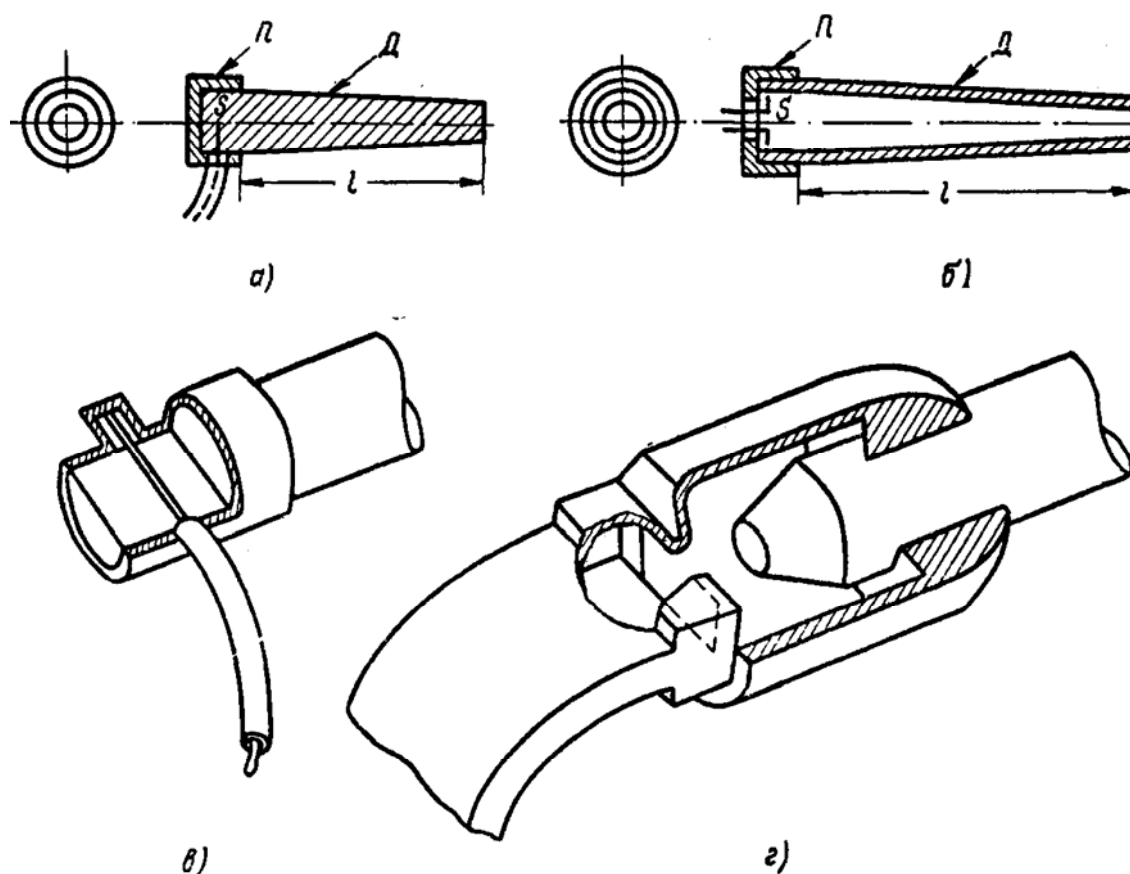
Рис. 8.1. Простые диэлектрические антенны: а – сплошная, б – полая (трубчатая), в – питание антенны с помощью коаксиального кабеля, г – возбуждение антенны посредством волновода
