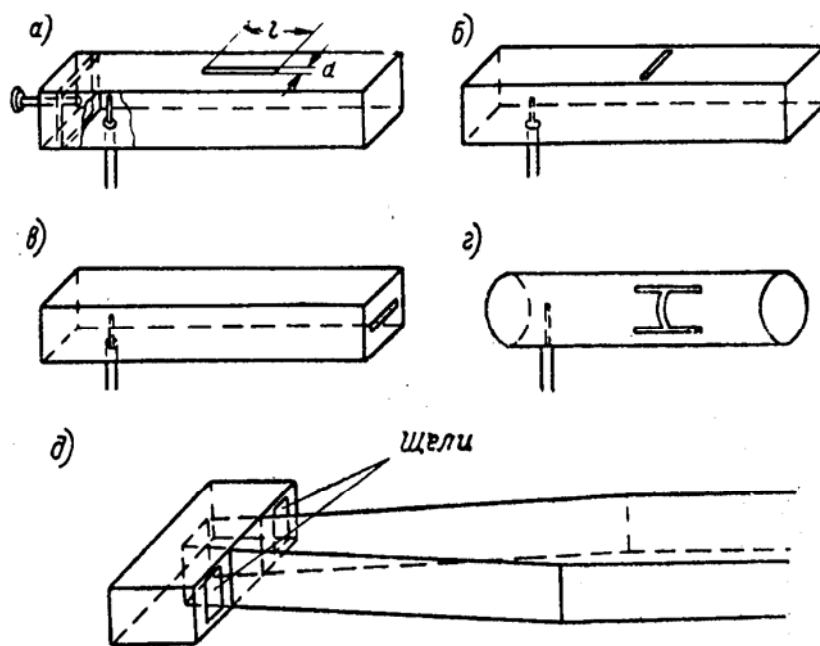
Рис. 6.1. Волноводные однощелевые антенны с использованием прямоугольного и круглого волноводов: а – продольная щель, б – поперечная щель, в – торцовая щель, г – H-образная щель, д – антенна обратного излучения
