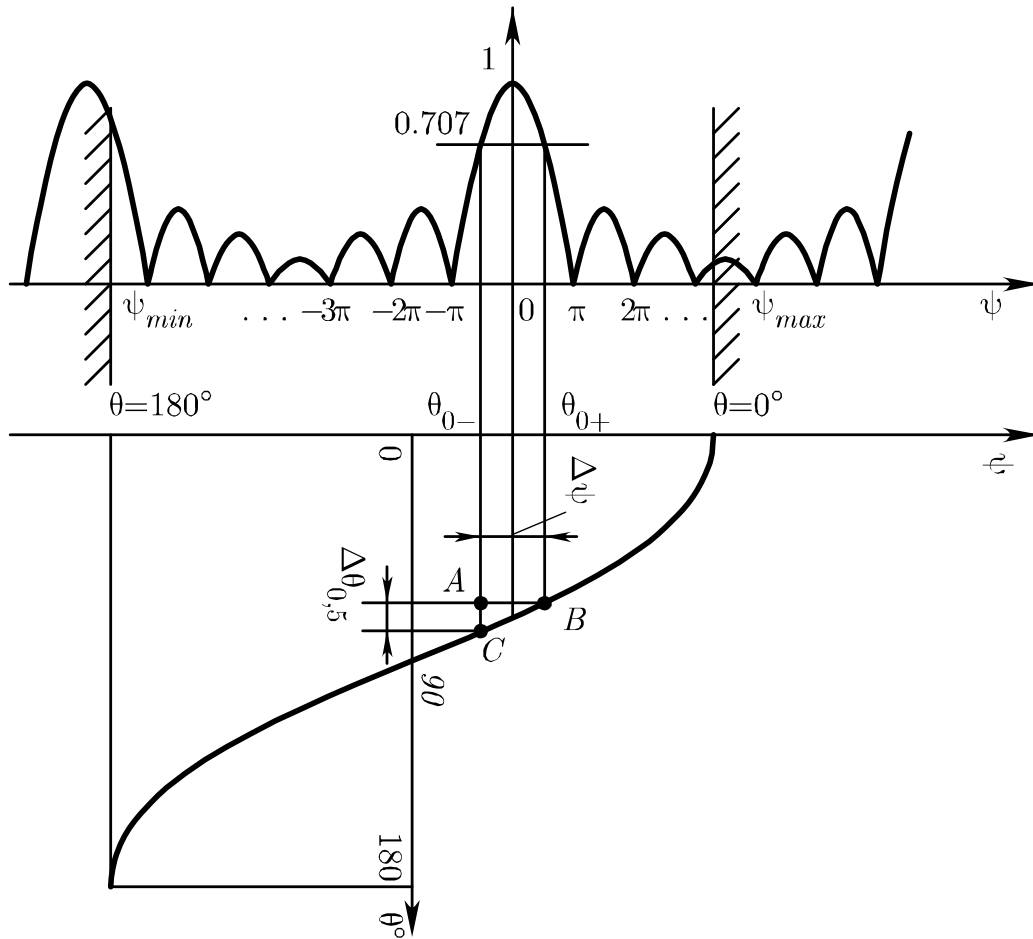
Рис. 9.5. Определение \Delta\theta_{0,5} по графику множителя комбинирования
