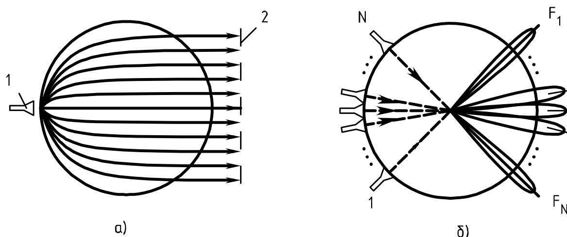
Рис. 10.6. Сферическая линза Лüneберга
