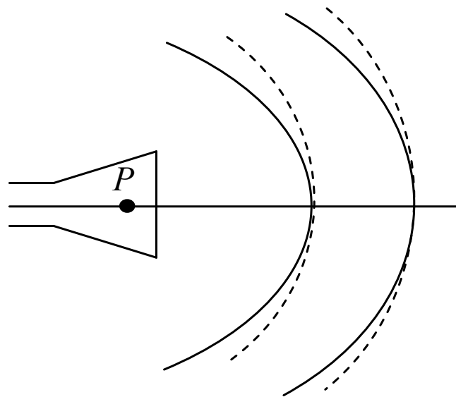
Рис. 1.4. Поверхности равных фаз у антенны, не имеющей фазового центра
