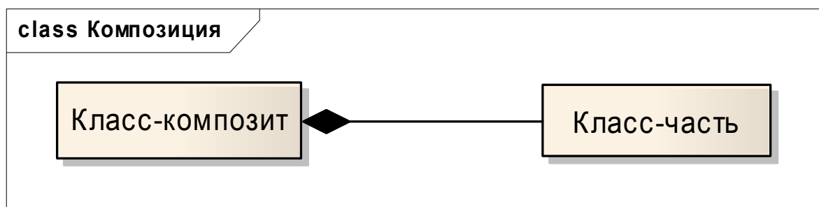
Рис. 2.18. Графическое изображение отношения композиции
