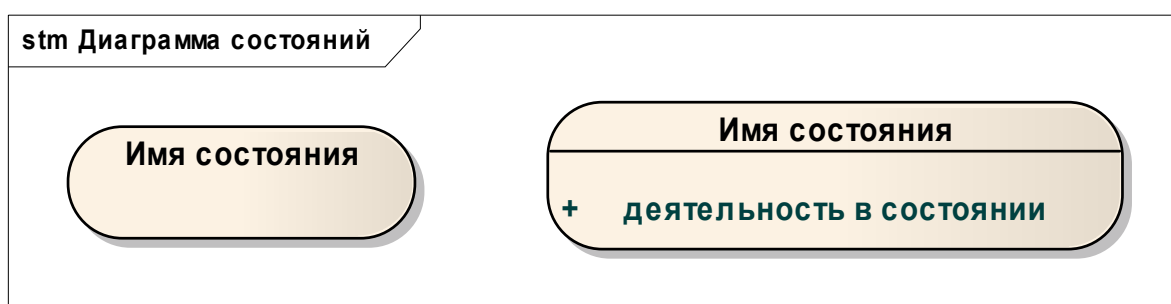
Рис. 3.3. Графическое изображение состояний
