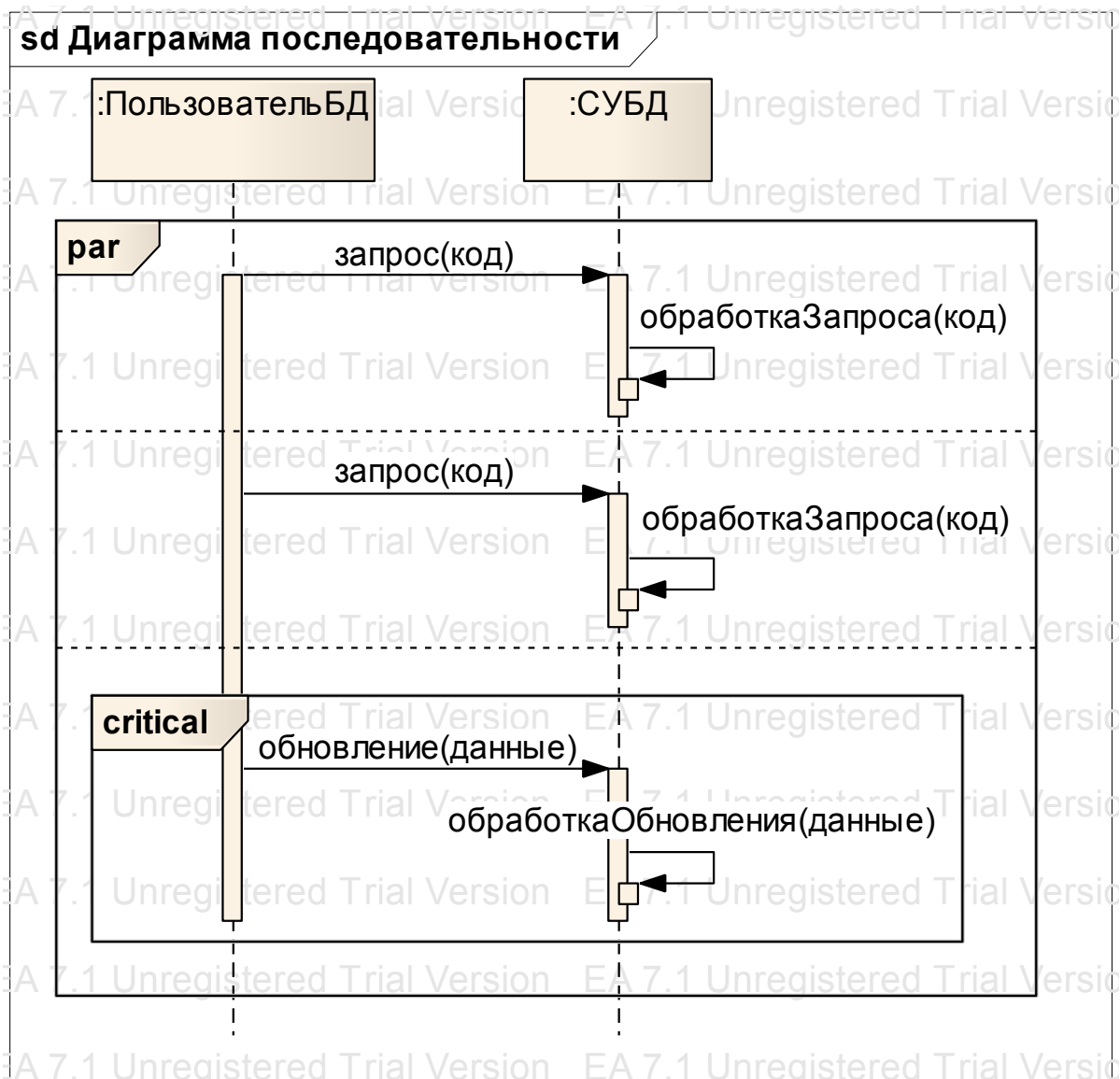
Рис. 4.21. Пример комбинированного фрагмента critical
