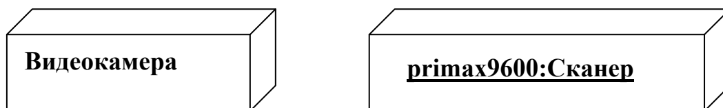
Рис. 5.10. Графическое изображение узла на диаграмме развертывания
