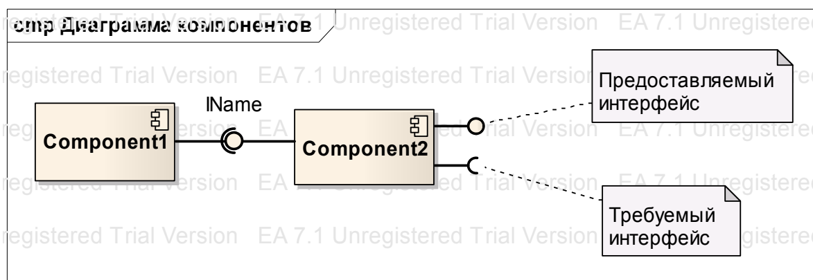
Рис. 5.8. Графическое изображение компонента с интерфейсами
