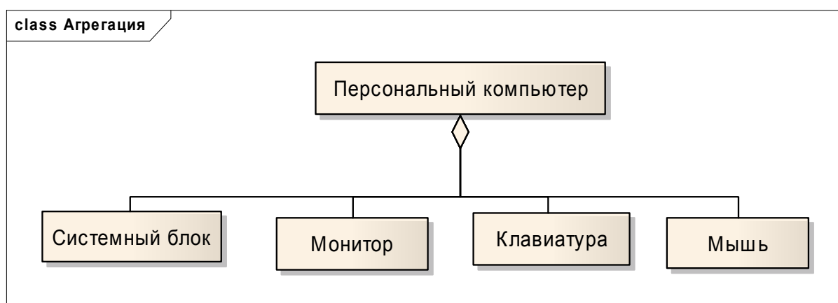
Рис. 2.17. Пример отношения агрегации.
