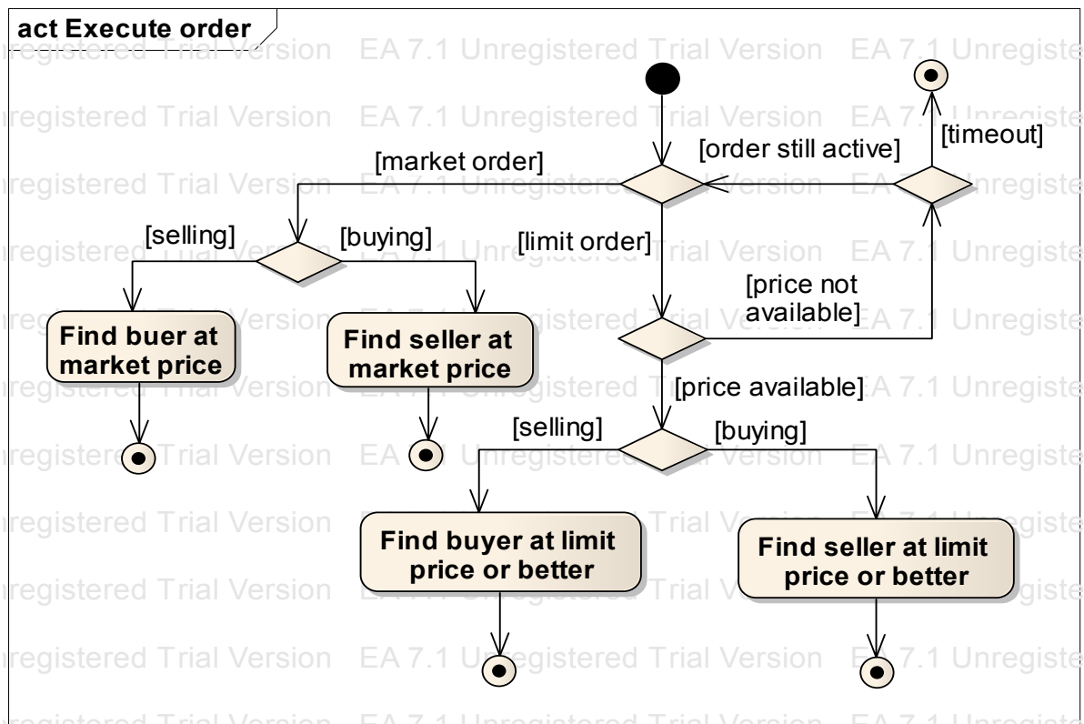
Рис. 4.27. Вложенная диаграмма деятельности для действия «Execute order»
