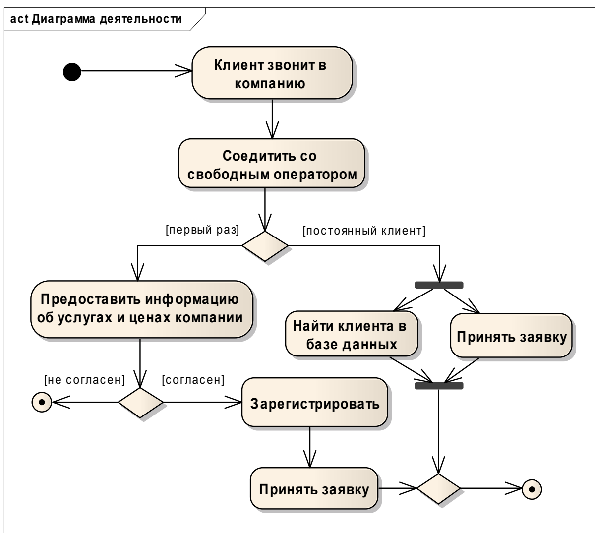
Рис. 4.22. Пример диаграммы деятельности
