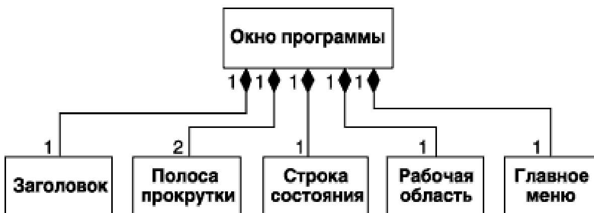
Рис. 2.19. Пример отношения композиции
