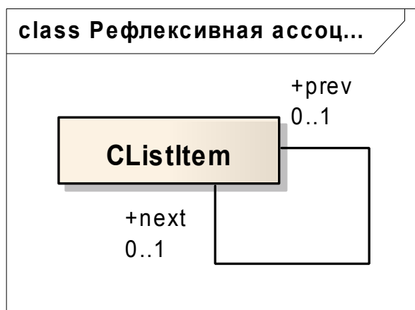
Рис. 2.8. Изображение рефлексивной ассоциации
