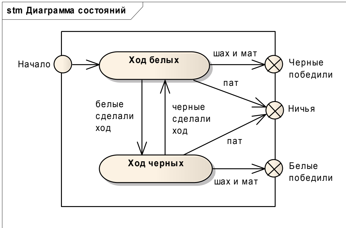
Рис. 3.9. Диаграмма состояний с точками входа и выхода
