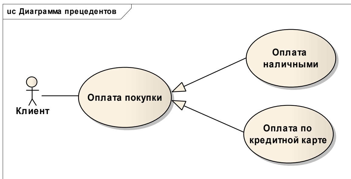
Рис. 4.8. Графическое изображение отношения обобщения
