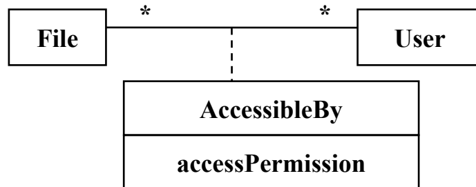
Рис. 2.11. Графическое изображение ассоциации-класса
