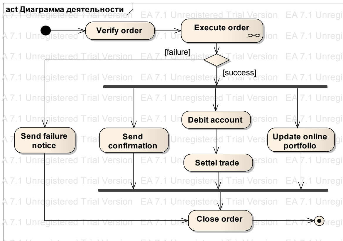
Рис. 4.26. Графическое изображение составной деятельности
