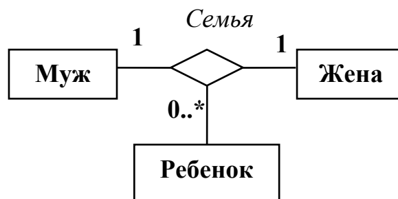
Рис. 2.10. Графическое изображение n -арной ассоциации
