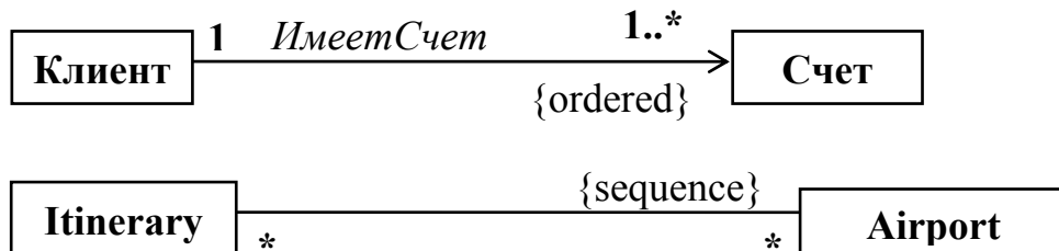
Рис. 2.9. Изображение ассоциации со строкой свойства
