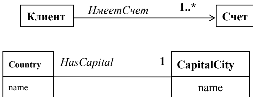
Рис. 2.6. Изображение кратности полюсов ассоциации
