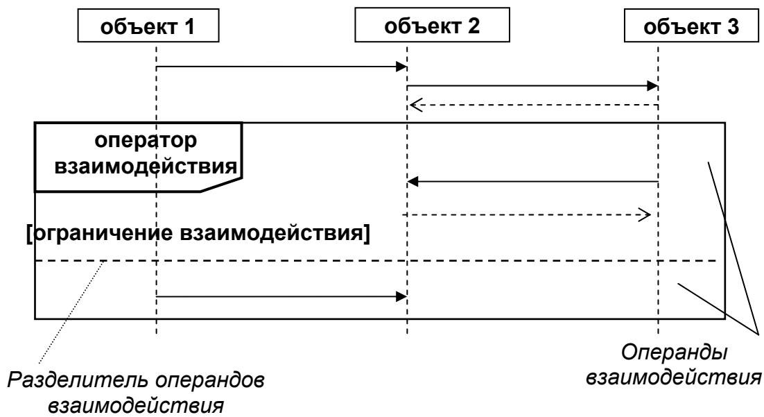
Рис. 4.16. Графическое изображение комбинированного фрагмента
