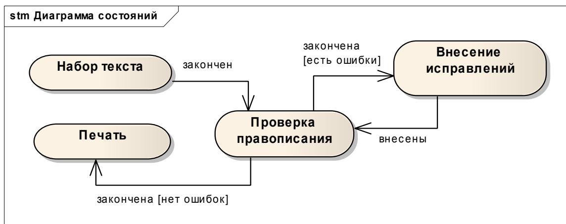
Рис. 3.6. Пример применения переходов со сторожевыми условиями
