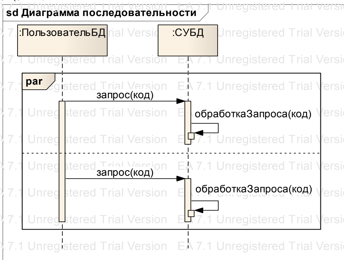
Рис. 4.20. Пример комбинированного фрагмента par
