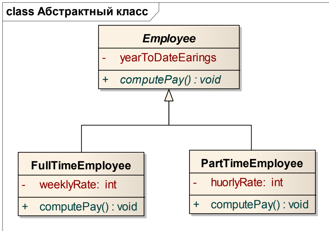
Рис. 2.14. Изображение абстрактного класса и абстрактной операции
