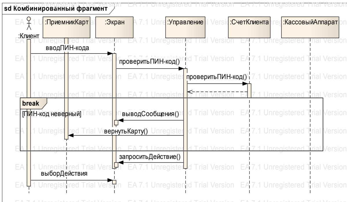
Рис. 4.16. Пример комбинированного фрагмента break
