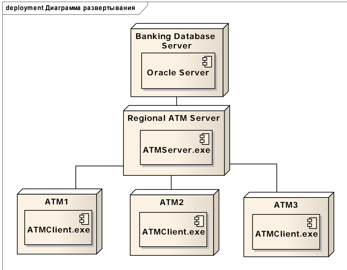
Рис. 5.13. Пример диаграммы развертывания
