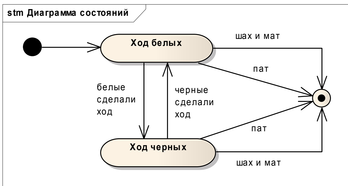
Рис. 3.8. Начальное и конечное состояния на диаграмме состояний
