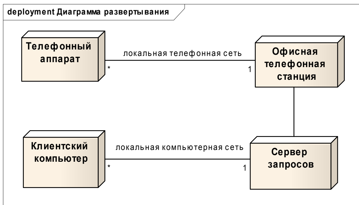
Рис. 5.11. Пути коммуникации между различными узлами
