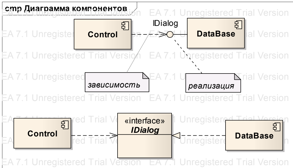
Рис. 5.7. Графическое изображение компонентов и связывающих их интерфейсов
