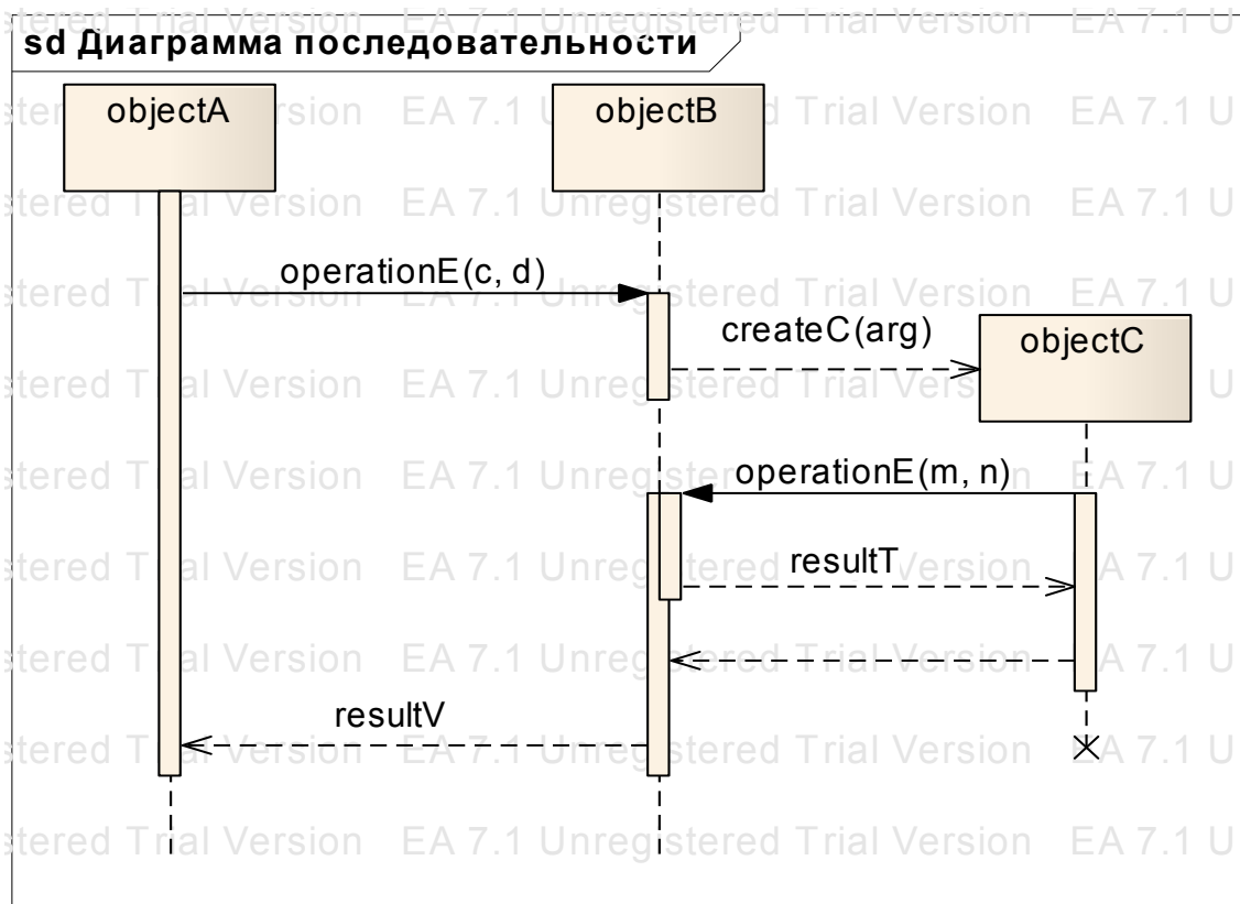
Рис. 4.14. Изображение сообщений с именем и списком аргументов
