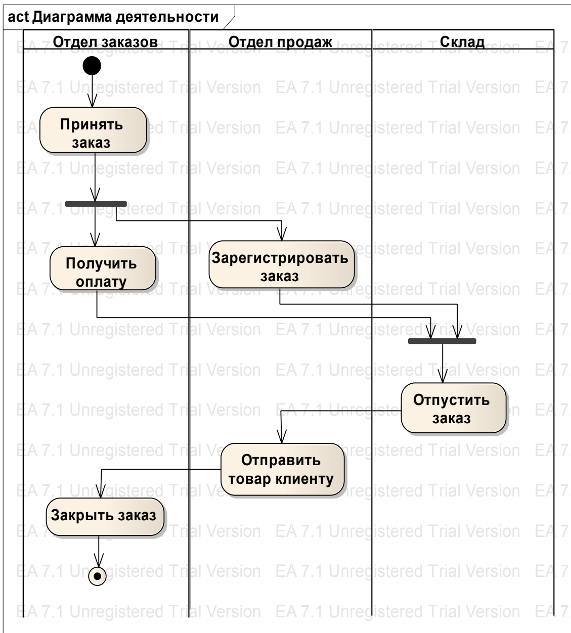
Рис. 4.28. Диаграмма деятельности с плавающими дорожками
