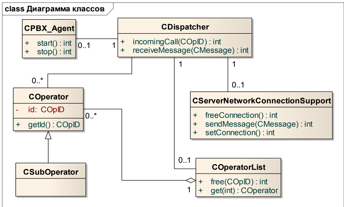
Рис. 2.1. Пример диаграммы классов (телефонная служба приема заявок, фрагмент)
