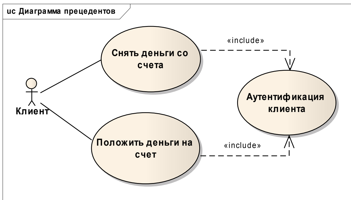
Рис. 4.5. Графическое изображение отношения включения
