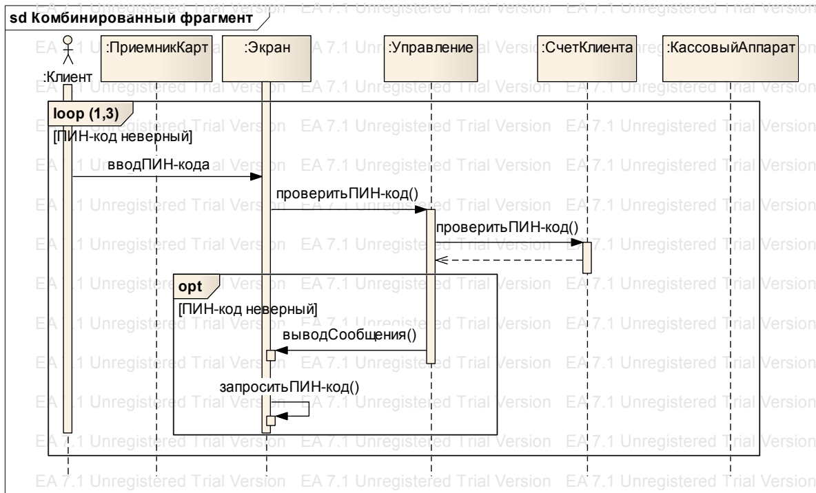
Рис. 4.19. Пример комбинированного фрагмента opt
