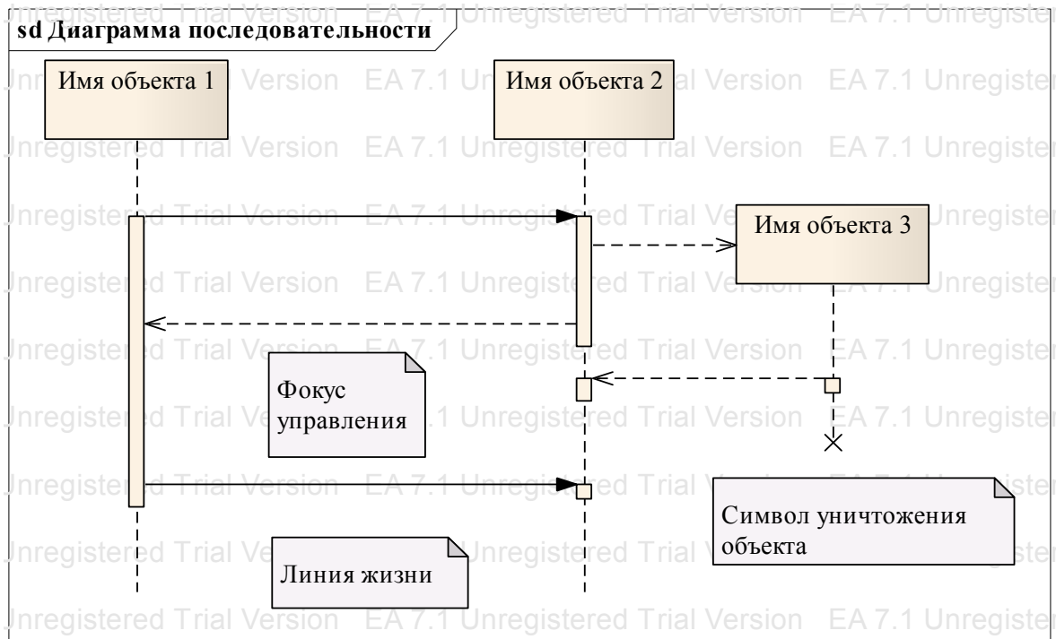
Рис. 4.11. Графические элементы диаграммы последовательности
