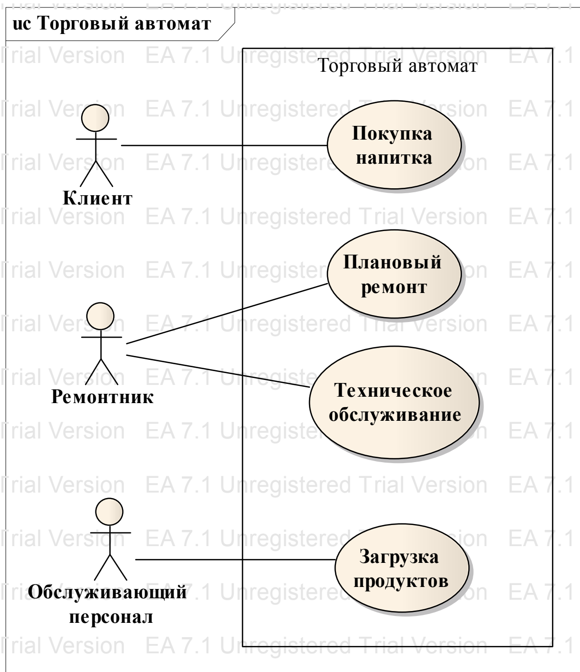
Рис. 4.4. Варианты использования торгового автомата
