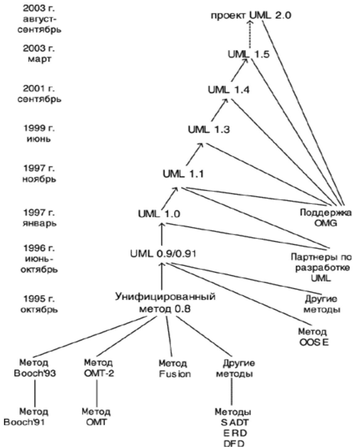
Рис. 1.1. Развитие языка UML
