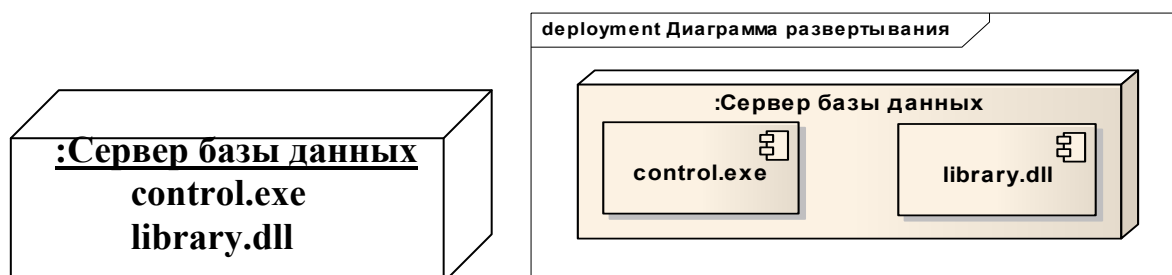
Рис. 5.12. Способы представления развертывания компонентов в узле
