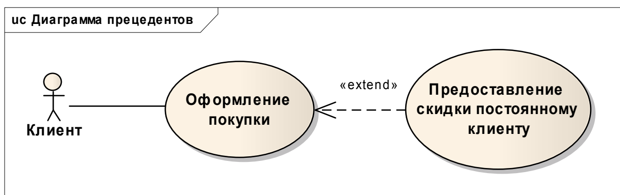
Рис. 4.6. Графическое изображение отношения расширения
