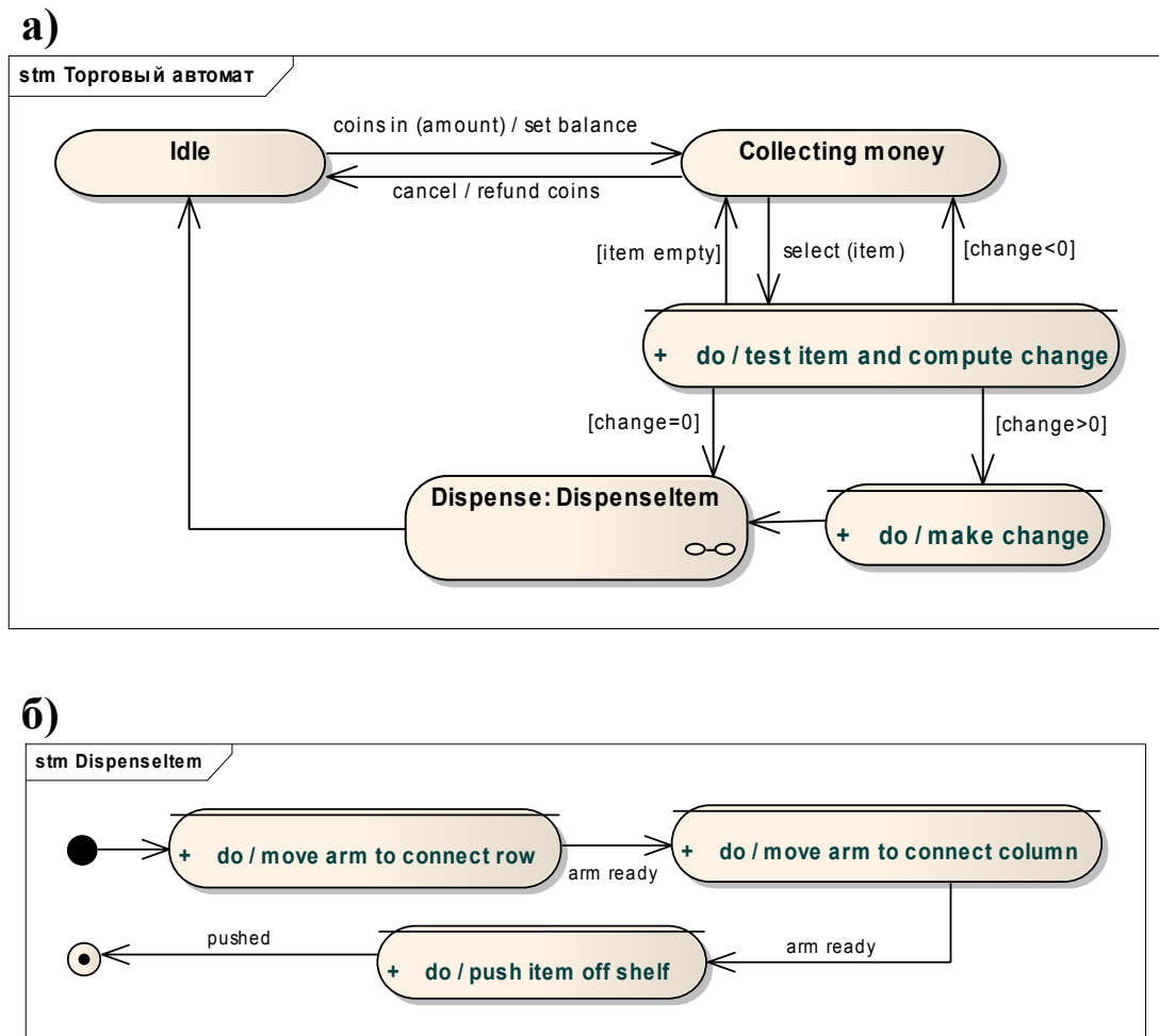
Рис. 3.15. Диаграмма состояний торгового автомата
