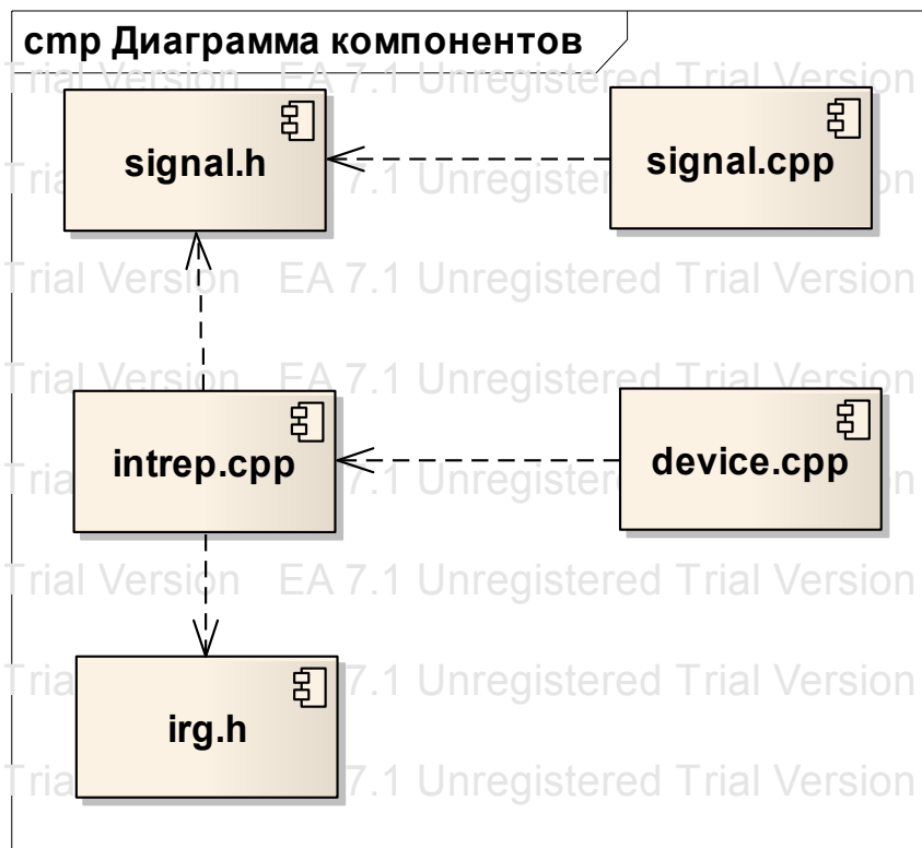
Рис. 5.4. Пример фрагмента диаграммы компонентов
