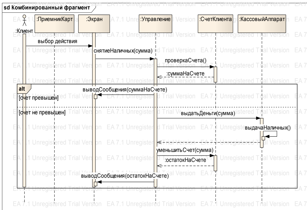
Рис. 4.18. Пример комбинированного фрагмента alt
