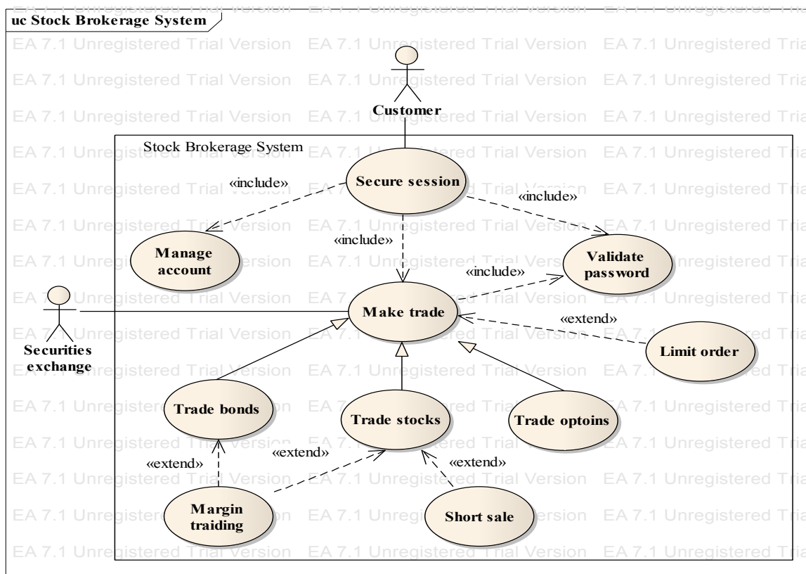
Рис. 4.1. Пример диаграммы вариантов использования (сетевая брокерская система)
