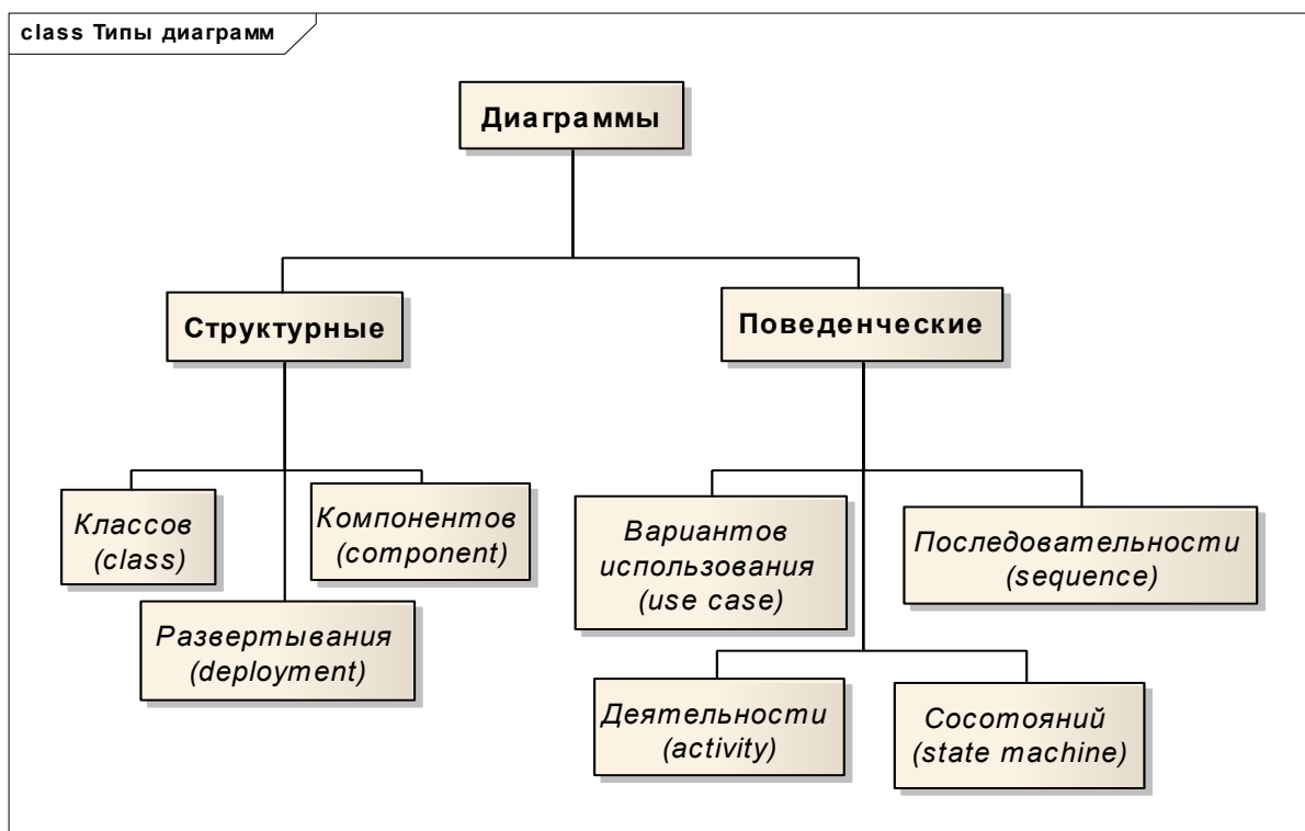
Рис. 1.2. Типы диаграмм языка UML
