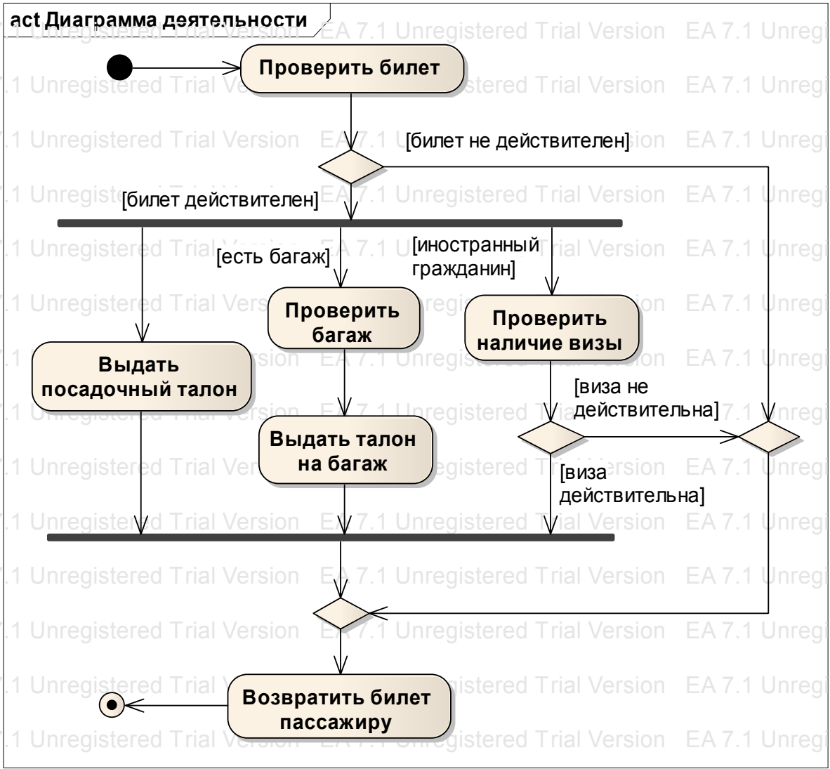
Рис. 4.25. Пример диаграммы деятельности для регистрации пассажиров
