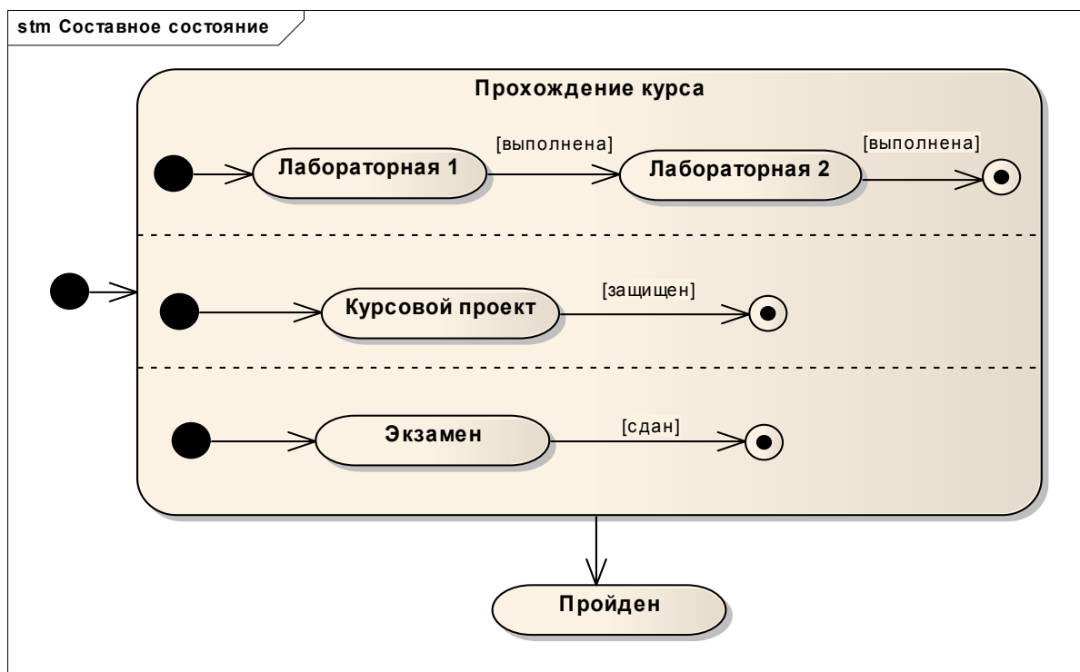
Рис. 3.13. Пример составного состояния с вложенными параллельными состояниями
