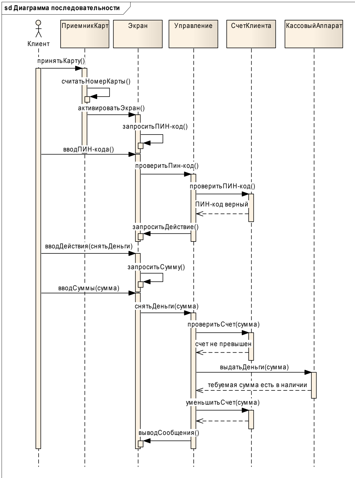
Рис. 4.10. Пример диаграммы последовательности (для основного потока событий варианта использования «Снятие денег через банкомат»)
