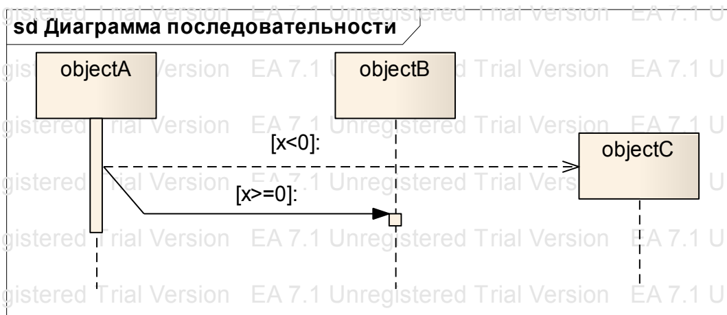
Рис. 4.15. Изображение ветвления потока управления
