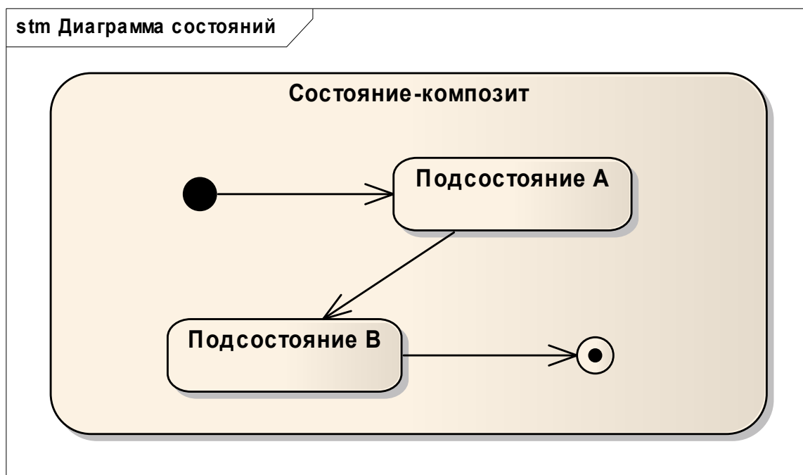
Рис. 3.10. Графическое представление составного состояния с последовательными подсостояниями
