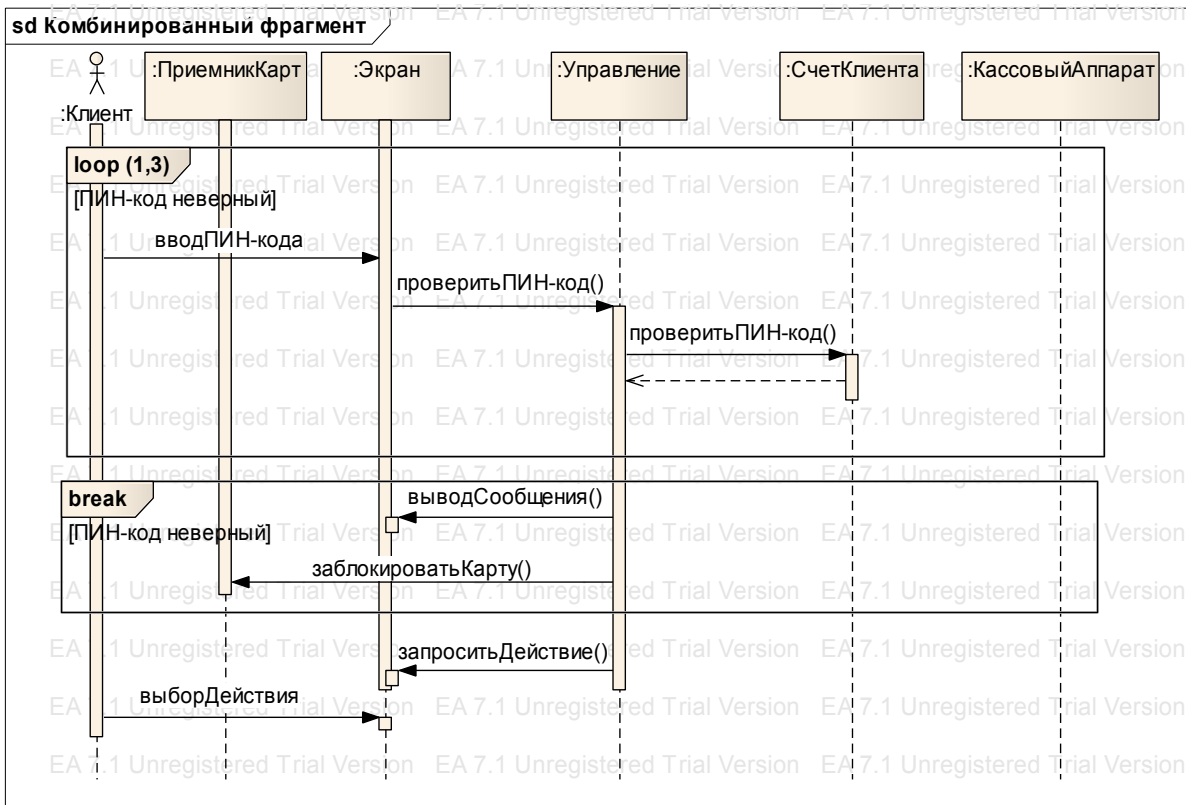
Рис. 4.17. Пример комбинированного фрагмента loop
