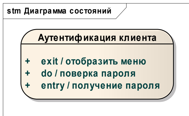
Рис. 3.4. Пример состояния с деятельностью
