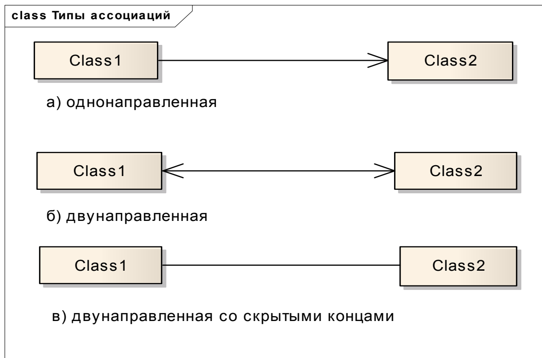
Рис. 2.4. Графическое изображение ассоциаций
