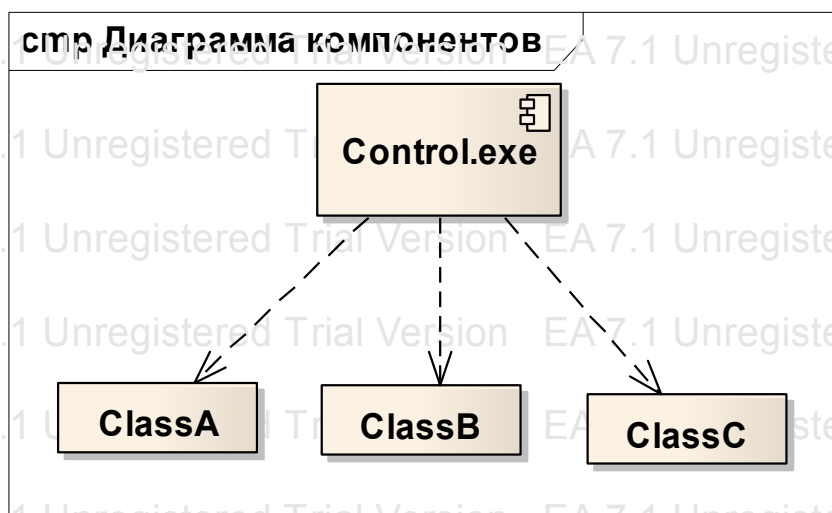
Рис. 5.5. Графическое изображение зависимости между компонентом и классами
